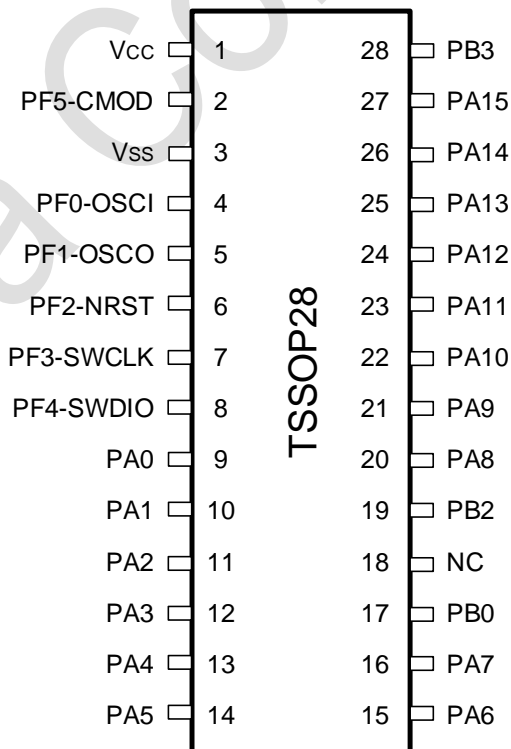
图 3-2 TSSOP28 Pinout4 PY32T020G4xP7-B (Top view)
