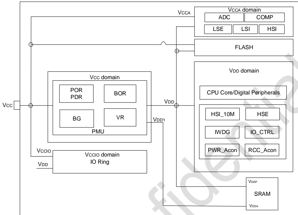
图 2-2 电源框图
